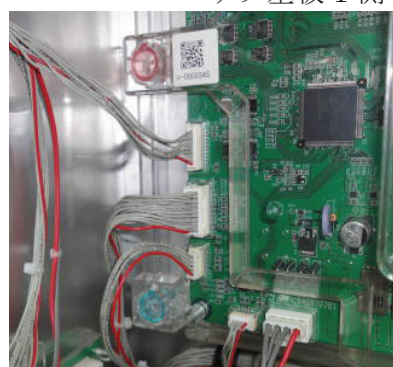
サブ基板1側
